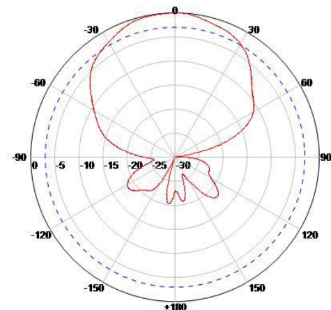
Вертикальная, 3 дБ
