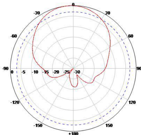
Горизонтальная, 3 дБ
